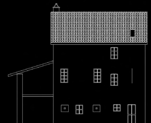
PROSPETTO B
