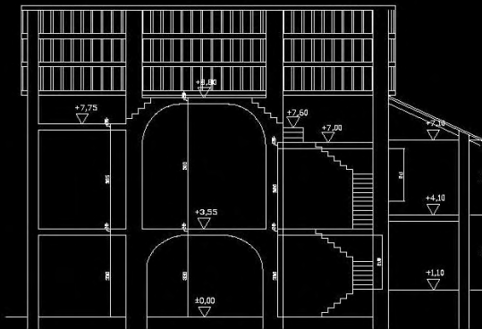
SEZIONE
