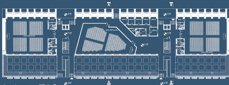
piano terreno - edificio C
